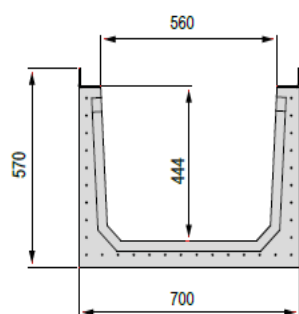
C700 folyóka:
