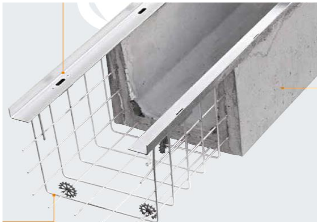
C600 folyóka:
