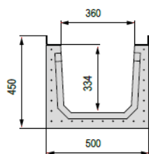
C700 folyóka:
